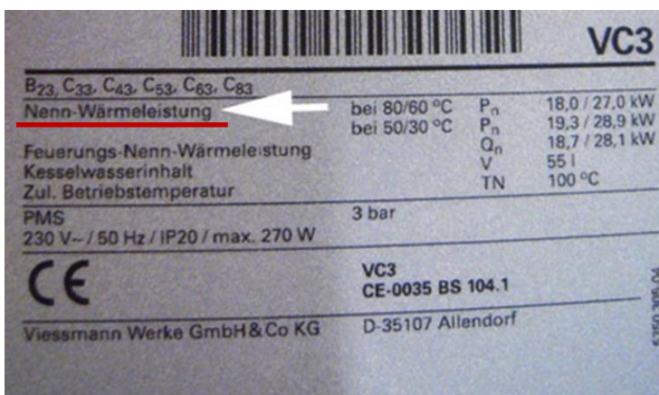
Beispiele für Typenschilder
